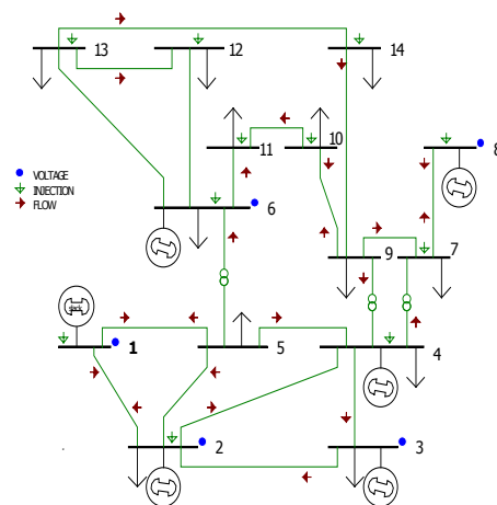
Figura 2: Sistema de 14 Barras IEEE con Distribución de las Mediciones
