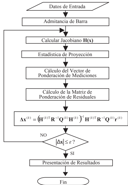
Figura 3: Diagrama de Flujo del Programa de Estimación Robusta
