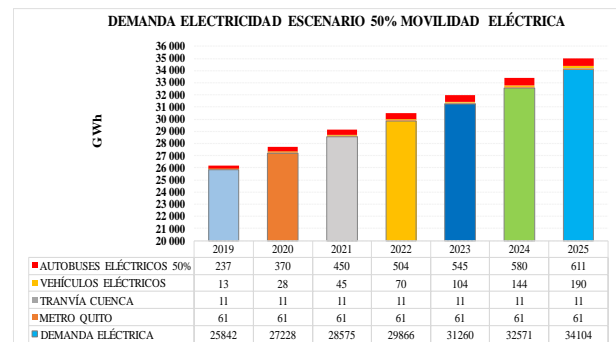
Figura 8: Demanda de Autobuses Eléctricos Escenario 2
