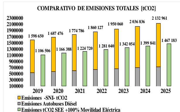
Figura 17: Emisiones Comparativas SNI + Autobuses Diésel versus Sistema de Movilidad Eléctrica
