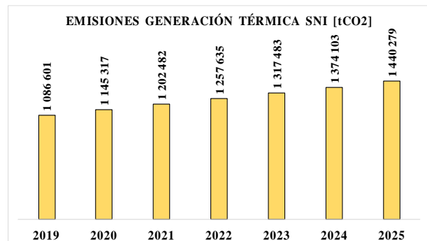
Figura 10: Emisiones Generación Térmica SNI, período 2019-2025
