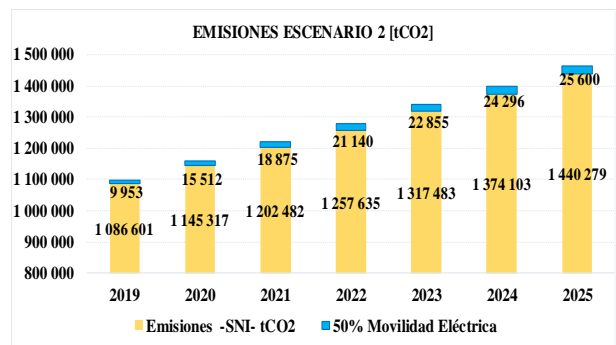
Figura 13: Emisiones Totales Toneladas CO 2 Escenario 2
