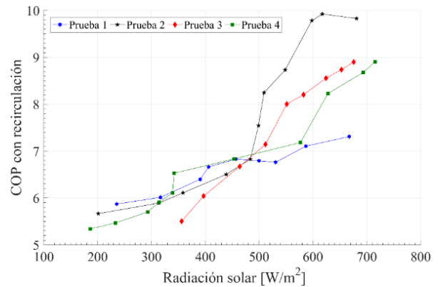
Figura 16. COP con recirculación vs. radiación solar
