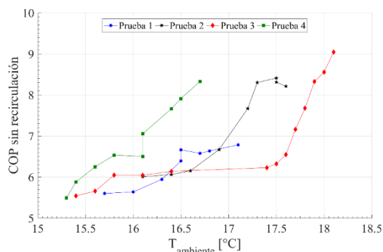
Figura 13. COP sin recirculación vs. temperatura ambiente
