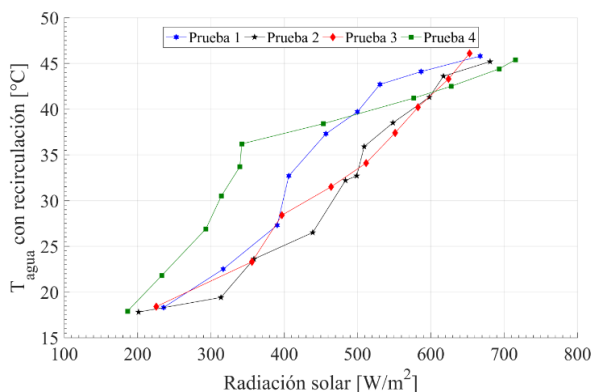
Figura 11. Temperatura del agua con configuración de recirculación vs. radiación solar
