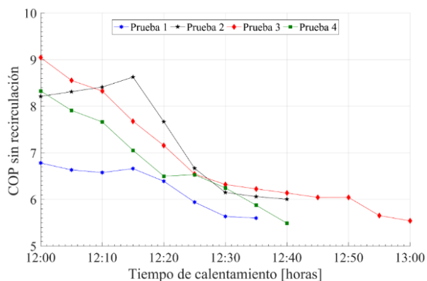
Figura 17. COP sin recirculación vs. tiempo de calentamiento
