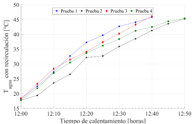
Figura 9. Incremento de la temperatura del agua con configuración de recirculación
