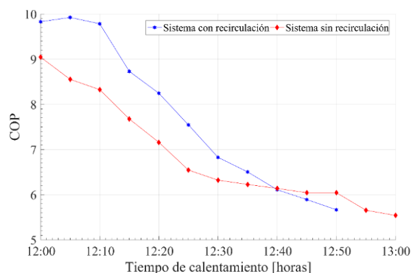
Figura 19. Comparativa del COP del sistema entre las configuraciones con recirculación y sin recirculación
