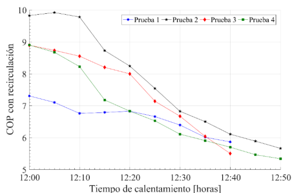
Figura 18. COP con recirculación vs. tiempo de calentamiento
