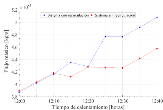
Figura 12. Flujo másico con recirculación y sin recirculación
