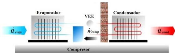
Figura 4. Ciclo de refrigeración por compresión de vapor [13]
