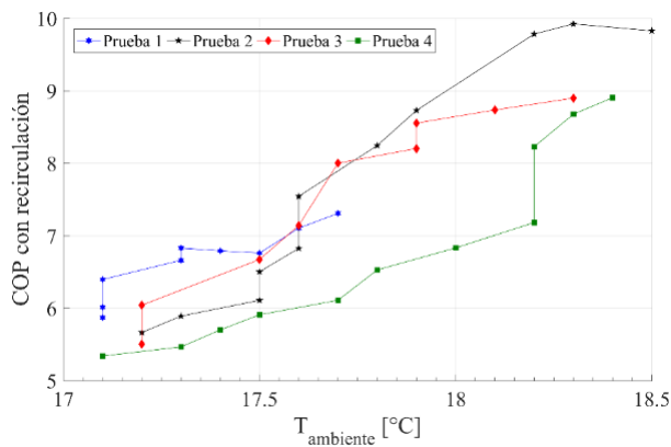
Figura 14. COP con recirculación vs. temperatura ambiente
