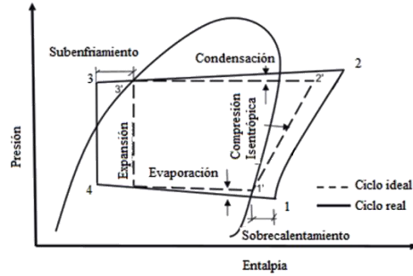
Figura 5. Diagrama P-h para el ciclo real de refrigeración por compresión de vapor [15]
