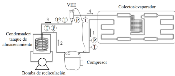
Figura 6. Componentes de un sistema DX-SAHP
