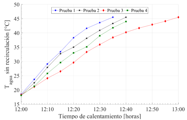
Figura 8. Incremento de temperatura del agua sin recirculación
