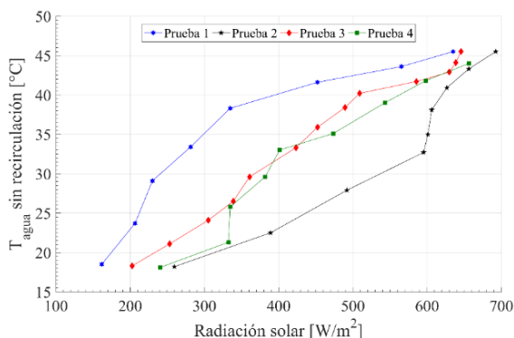
Figura 10. Temperatura del agua sin configuración de recirculación vs. radiación solar
