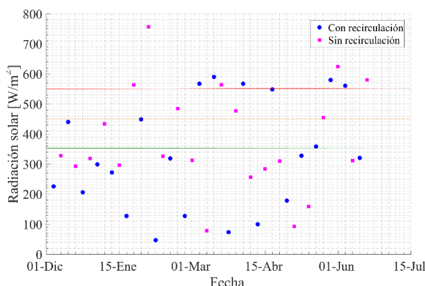
Figura 7. Valores promedio de radiación solar de días de prueba
