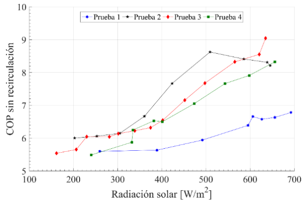
Figura 15. COP sin recirculación vs. radiación solar
