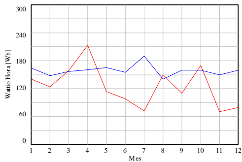
Figura 16: Comportamiento en consumo eléctrico simulado y medido
