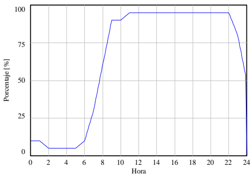
Figura 12: Curva de Distribución para iluminación
