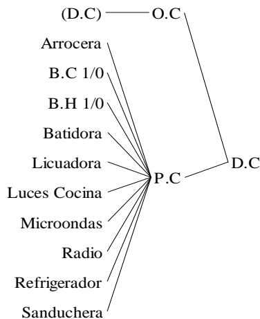
Figura 5: Consumo eléctrico en el cuarto de cocina
