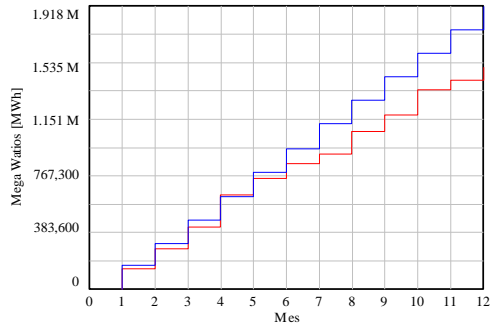
Figura 15: Consumo mensual acumulado estimado y medido
