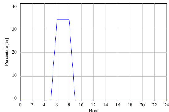
Figura 10: Curva de Distribución - Ducha
