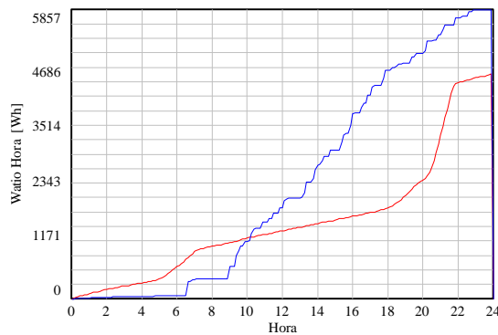
Figura 14: Consumo diario acumulado simulado y medido
