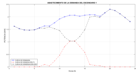
Figura 11: Abastecimiento de la demanda con la inclusión de generación FV en el escenario 1
