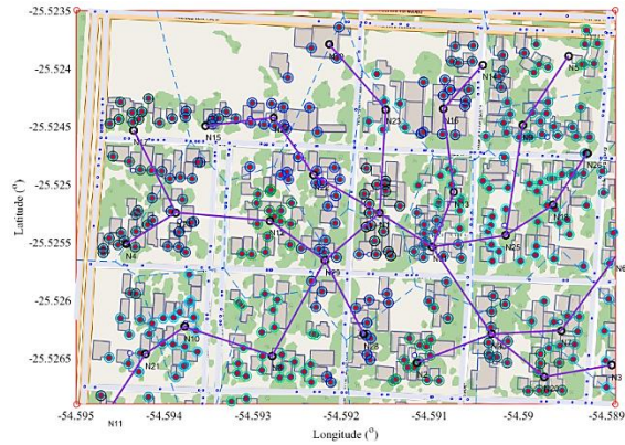
Figura 7: Escenario generado 3
