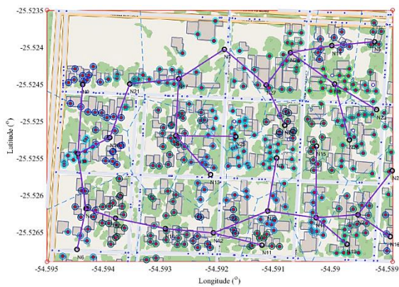
Figura 5: Escenario generado 1
