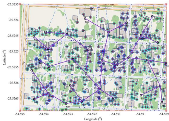
Figura 6: Escenario generado 2
