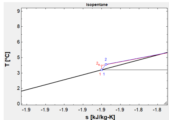
Figura 6: Determinación de la potencia teórica y real con isopentano. Detalle 2,2
