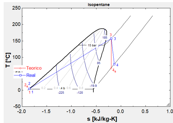
Figura 5: Determinación de la potencia teórica y real con isopentano
