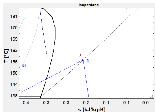
Figura 7: Determinación de la potencia teórica y real con isopentano. Detalle 3,3
