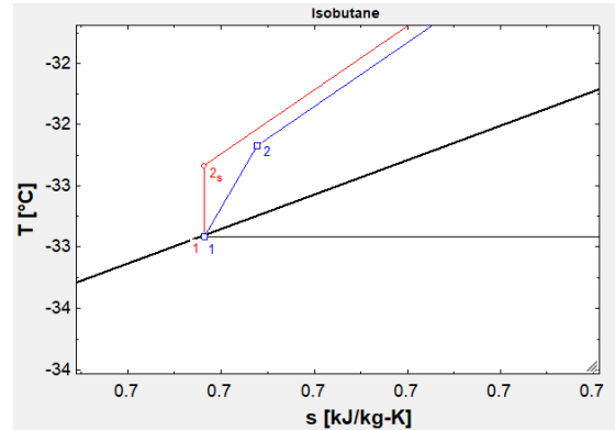
Figura 9: Determinación de la potencia teórica y real con isobutano. Detalle 2,2
