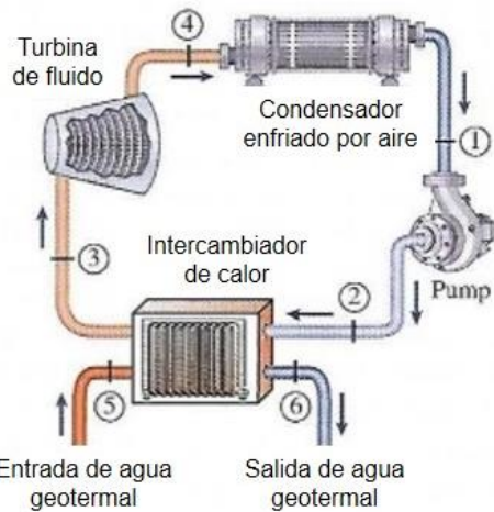
Figura 1: Diseño general de la central geotérmica (Y. Cengel & M. Boles 8va edición)
