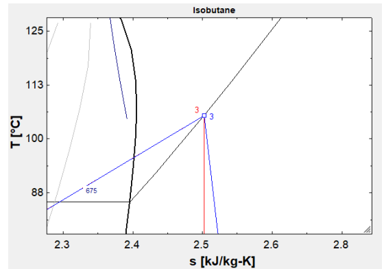
Figura 10: Determinación de la potencia teórica y real con isobutano. Detalle 3,3
