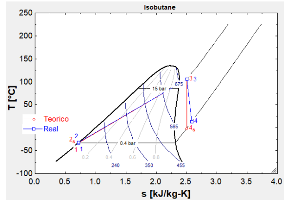
Figura 8: Determinación de la potencia teórica y real con isobutano
